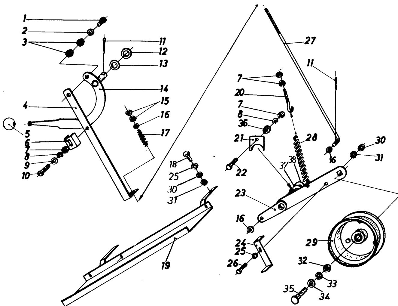
SCHAKELSYSTEEM MAAIBORD FEED TABLE CLUTCH LEVER DISPOSITIF D'ACCOUPLEMENT TABLIER HANDHEBEL PLATTFORMEINRÜCKUNG
